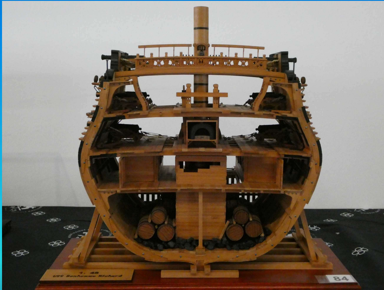
SEZIONE MAESTRA BONHOMME RICHARD
